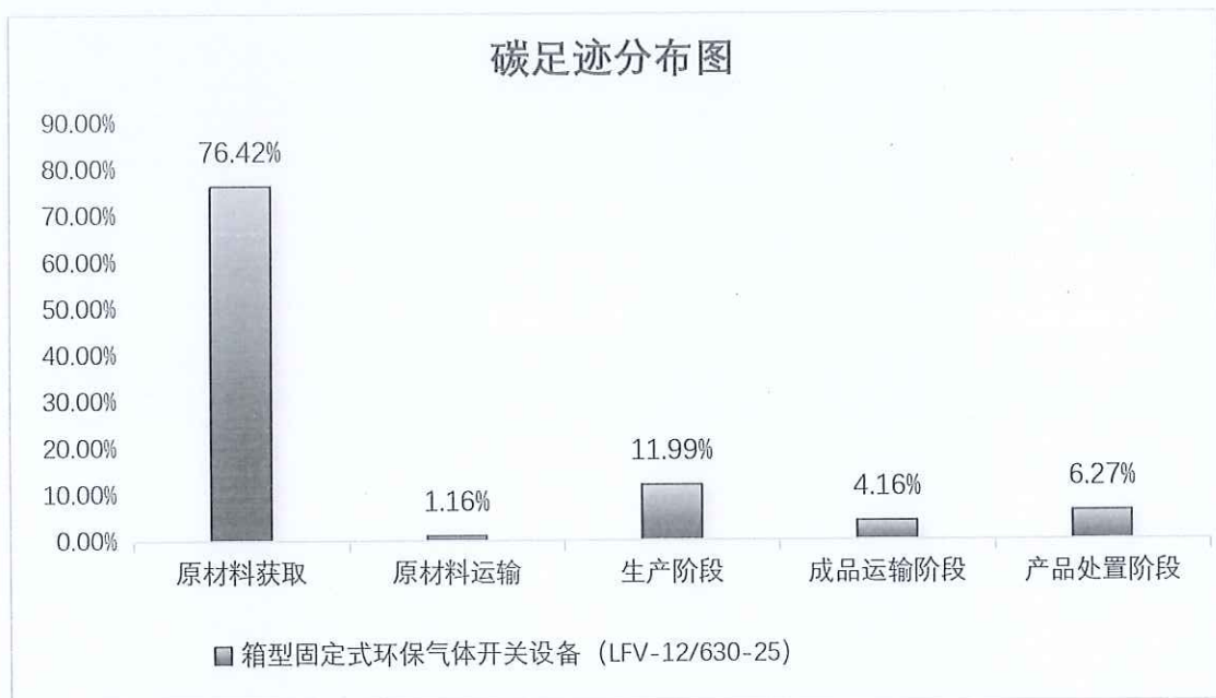
图 5.2.1.2 箱型固定式环保气体开关设备 (LFV-12/630-25) 生命周期阶段碳排放分布图
