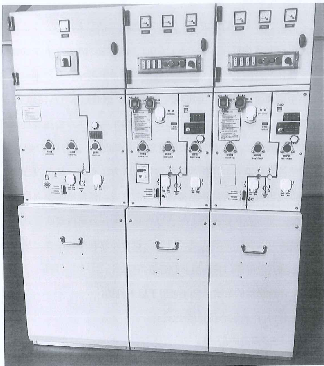
环保型全绝缘全密封交流金属环网开关设备 (LGXGN-12V/630-20)
