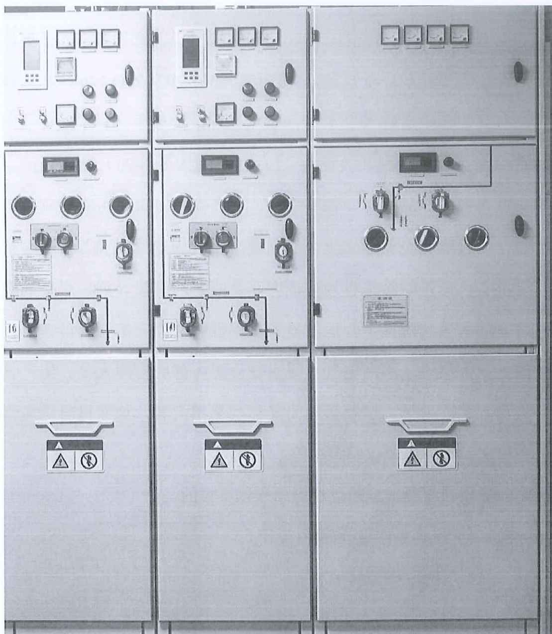
固体绝缘交流金属环网开关设备 (LGGT10-12V/630-20)
