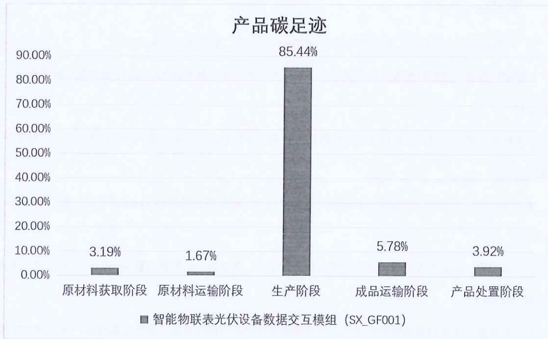
图 5.2.2 智能物联表光伏设备数据交互模组 (SX_GF001) 生命周期阶段碳排放分布图
