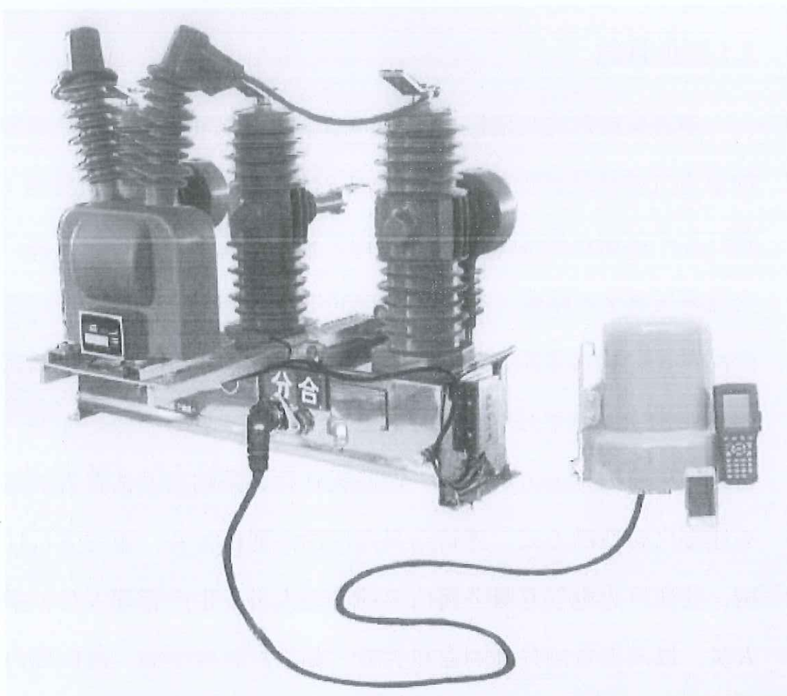
户外交流高压真空断路器 (ZW32-12/T630-20)
