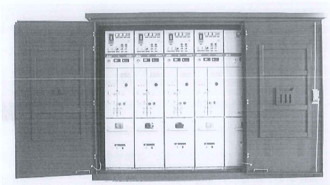
预装式封闭环网箱 (JLHXGW-12)
