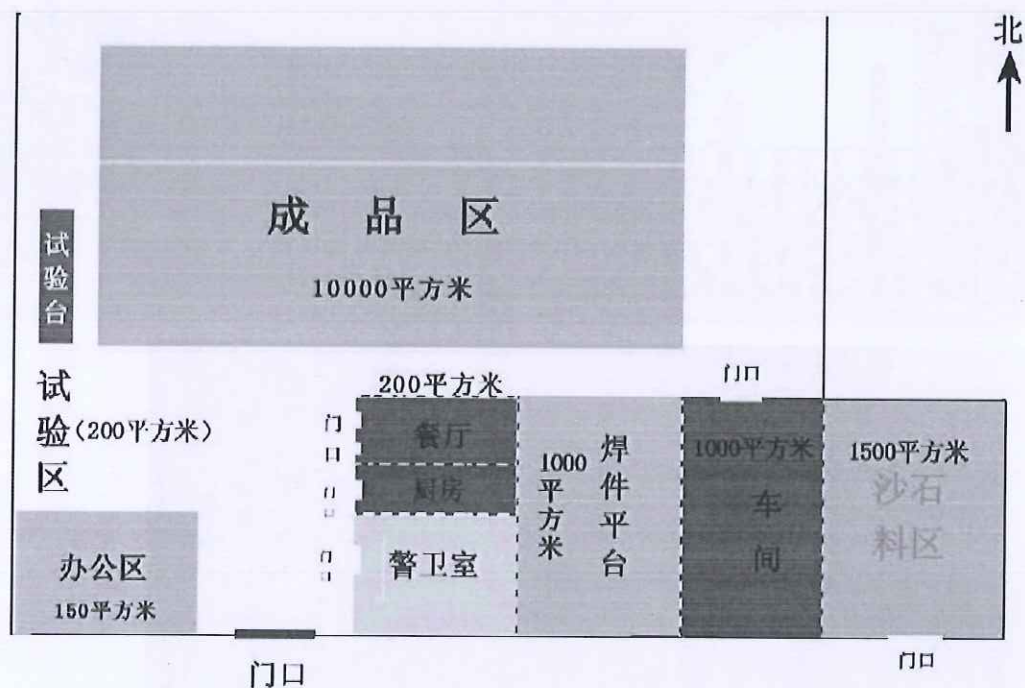
河北富联电气设备有限公司厂区平面图
