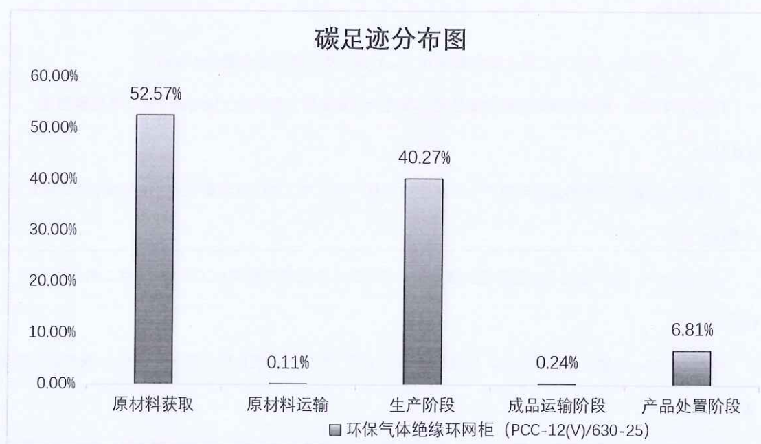
图 5.2.1.2 环保气体绝缘环网柜 (PCC-12(V)/630-25) 生命周期阶段碳排放分布图
