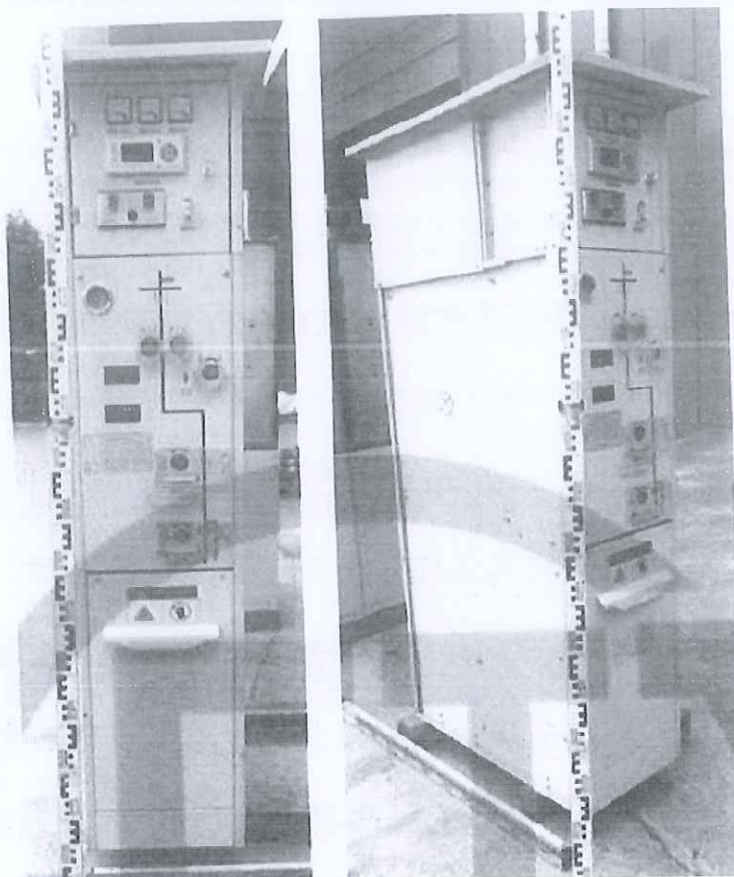
环保气体绝缘环网柜 (PCC-12(V)/630-25)
