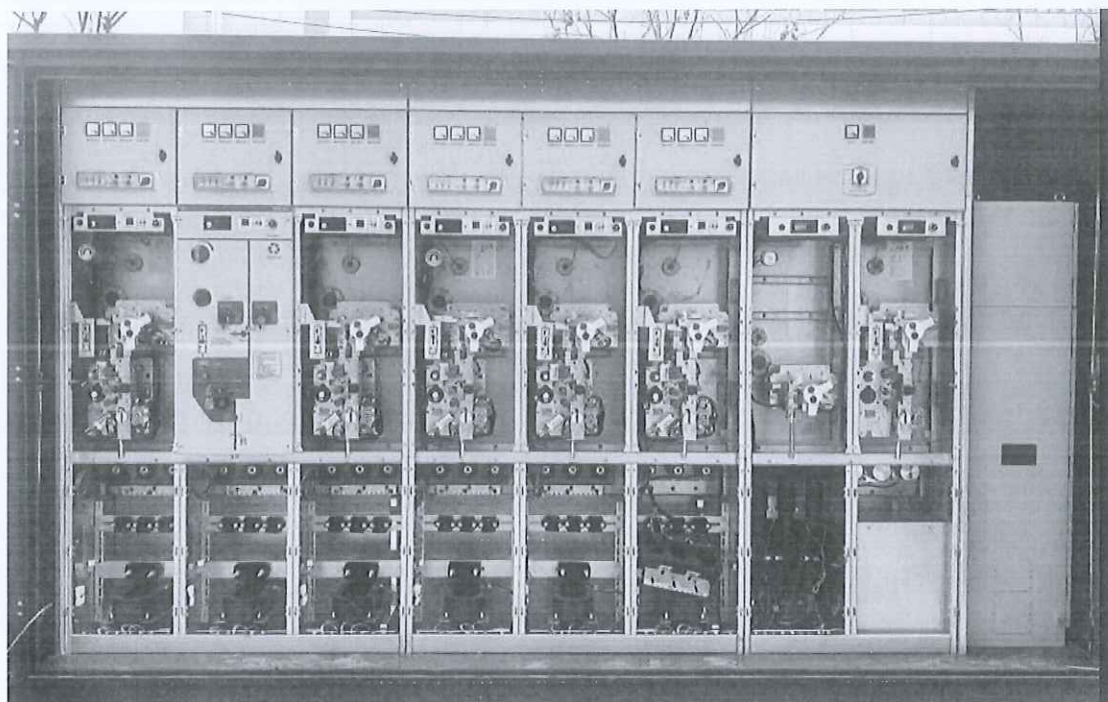
环网箱（箱式开闭所）（HXGW-12）
