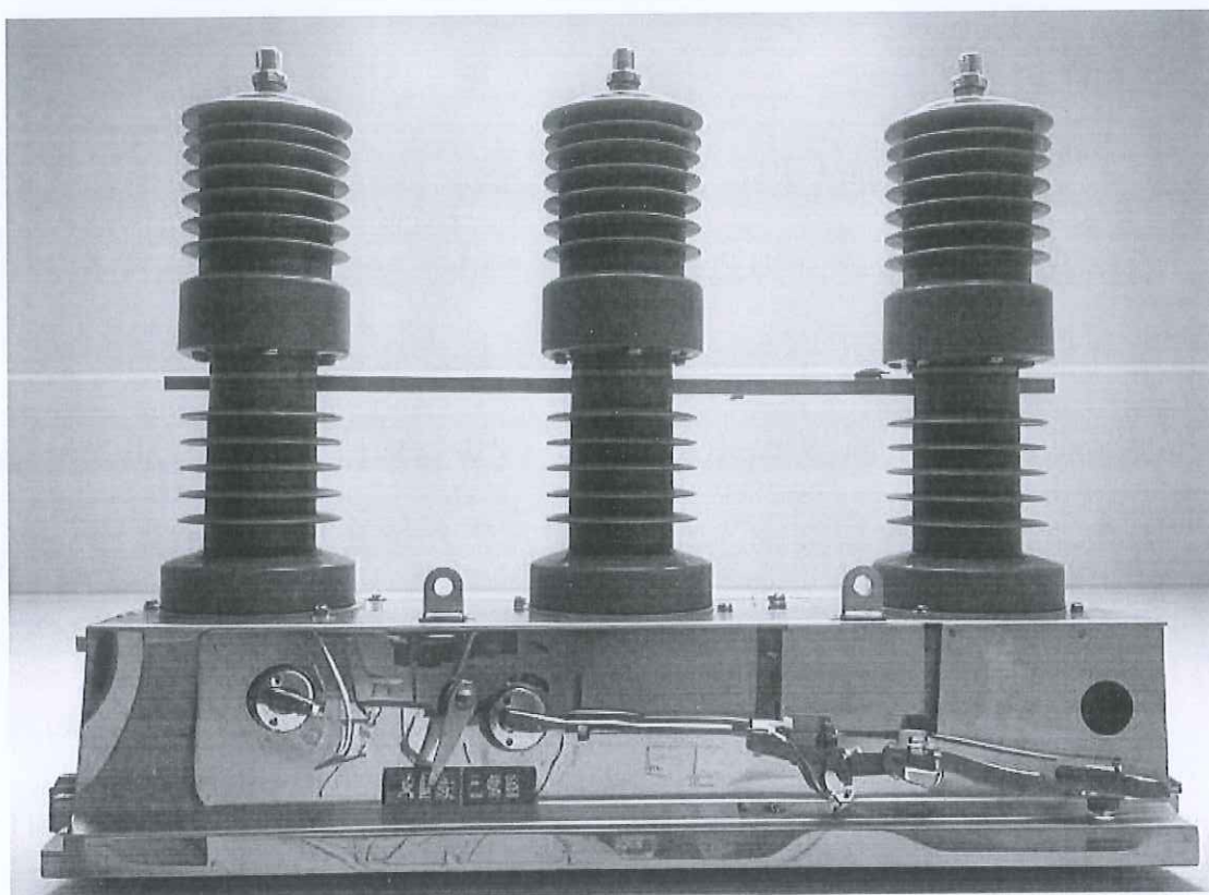
一二次融合成套柱上断路器(电容取电) (ZW32S-12/630-25)
