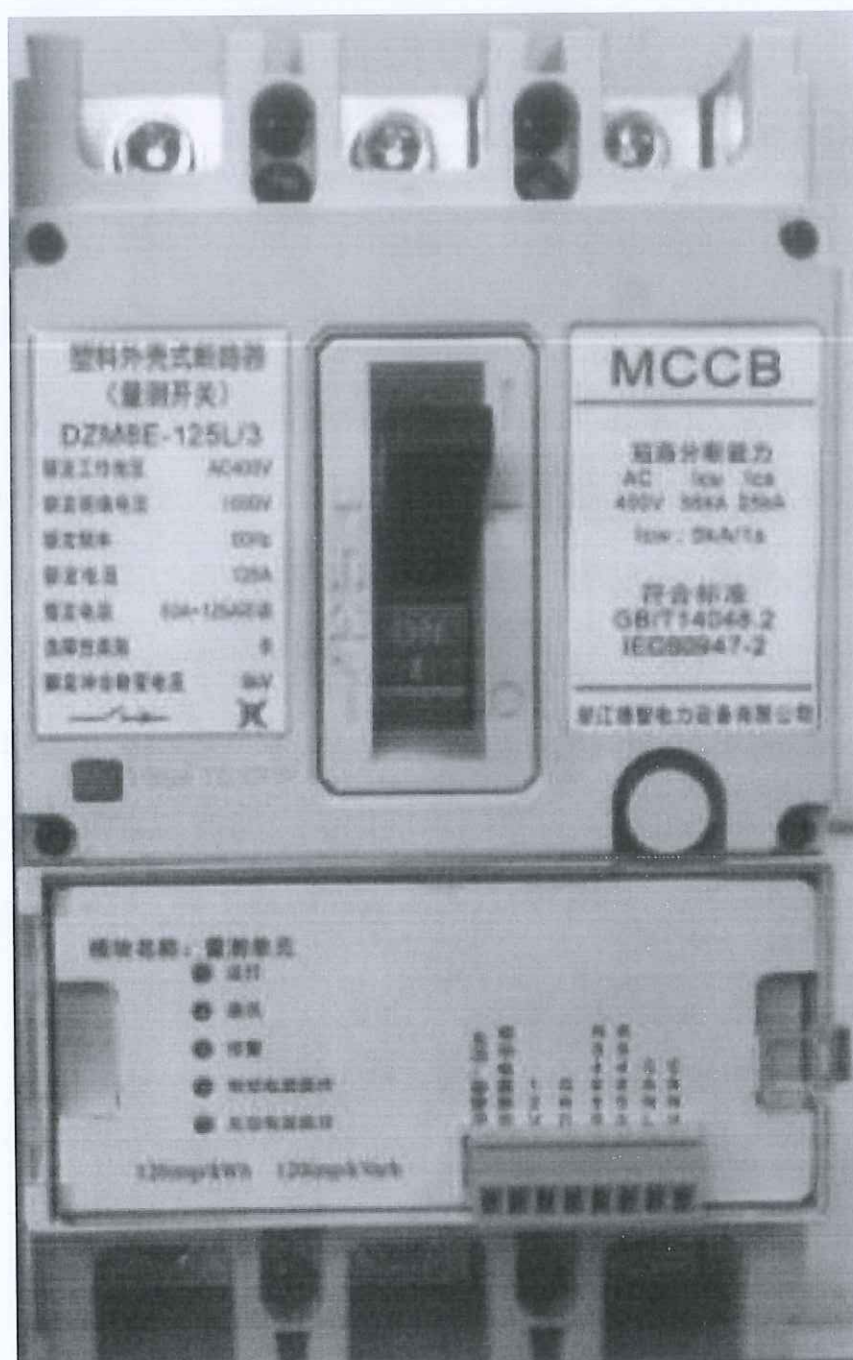
塑料外壳式断路器（量测开关）（DZM8E-250L/3）
