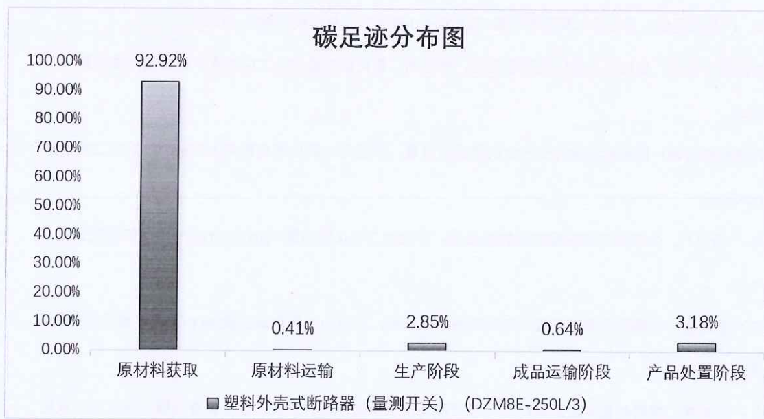
图 5.2.1.2 塑料外壳式断路器（量测开关）（DZM8E-250L/3）生命周期阶段碳排放分布图
