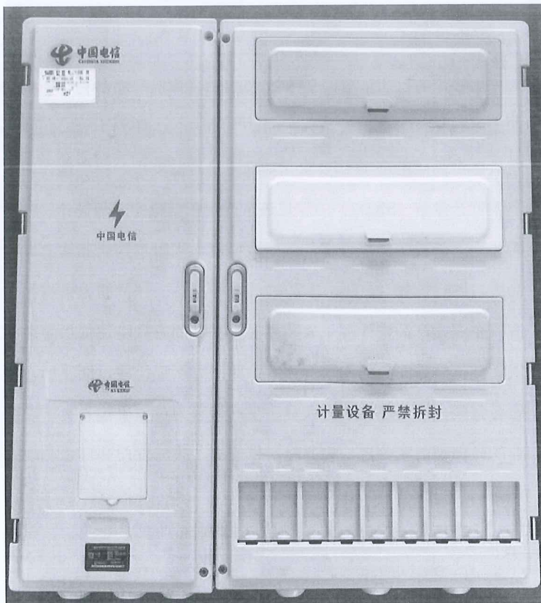
单相多表位计量箱 (SXD2)
