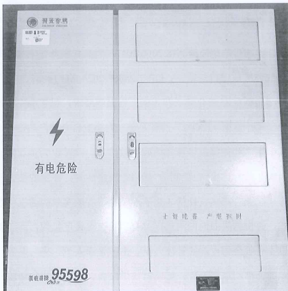
单相多表位金属计量箱 (BXD2)
