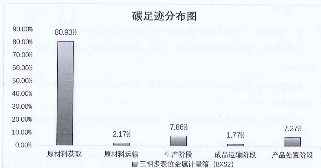
图 5.2.1.2 三相多表位金属计量箱 (BXS2) 生命周期阶段碳排放分布图
