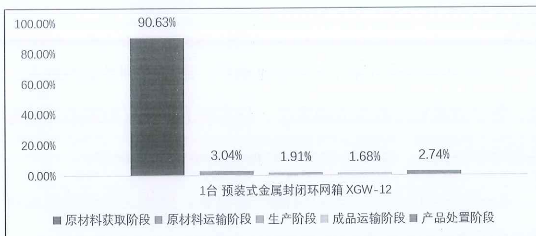
图 5.2-2-3 1 台 预装式金属封闭网箱 XGW-12 生命周期阶段碳排放分布图
