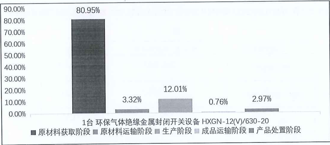
图 5.2-2-1 1 台 环保气体绝缘金属封闭开关设备 HXGN-12(V)/630-20 生命周期阶段碳排放分布图
