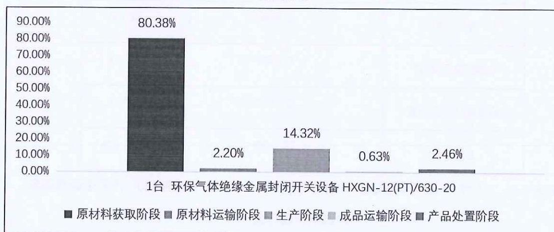
图 5.2-2-2 1 台 环保气体绝缘金属封闭开关设备 HXGN-12(PT)/630-20 生命周期阶段碳排放分布图
