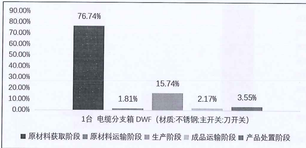
图 5.2-2-2 1 台 电缆分支箱 DWF (材质:不锈钢;主开关:刀开关) 生命周期阶段碳排放分布图
