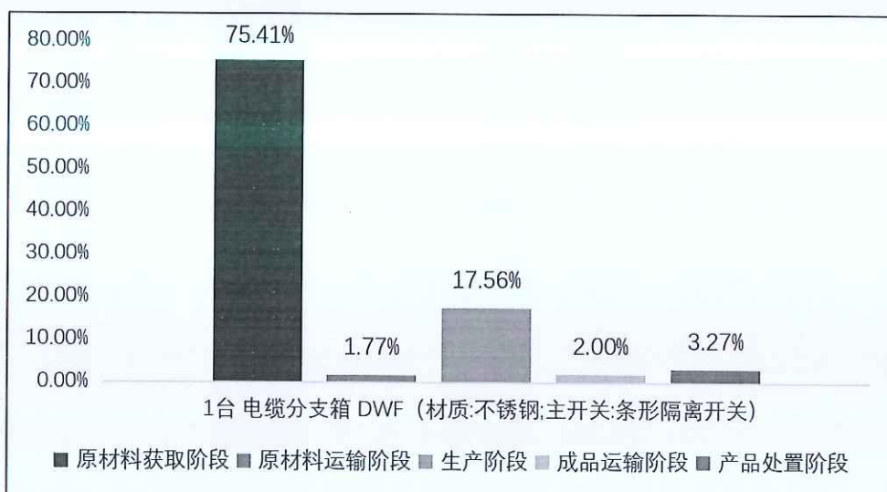
图 5.2-2-3 1 台 电缆分支箱 DWF (材质:不锈钢;主开关:条形隔离开关) 生命周期阶段碳排放
