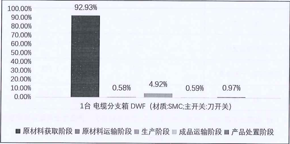
图 5.2-2-5 1 台 电缆分支箱 DWF（材质:SMC;主开关:刀开关） 生命周期阶段碳排放分布图
