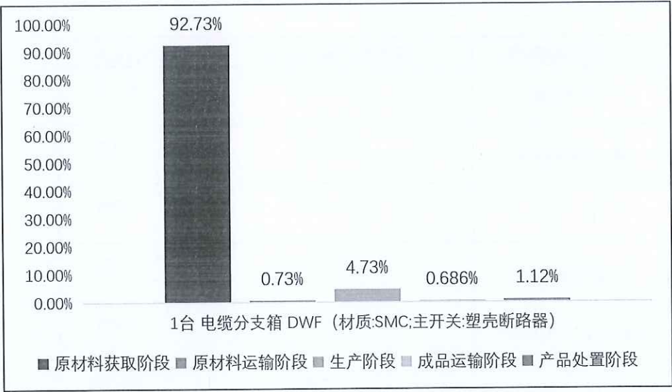
图 5.2-2-4 1 台 电缆分支箱 DWF（材质:SMC;主开关:塑壳断路器） 生命周期阶段碳排放分布图
