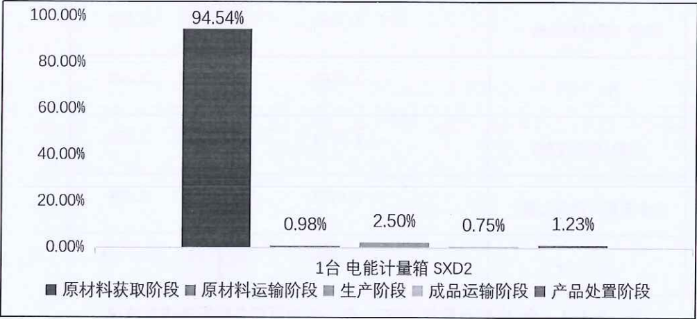
图 5.2-2-4 1 台 电能计量箱 SXD2 生命周期阶段碳排放分布图
