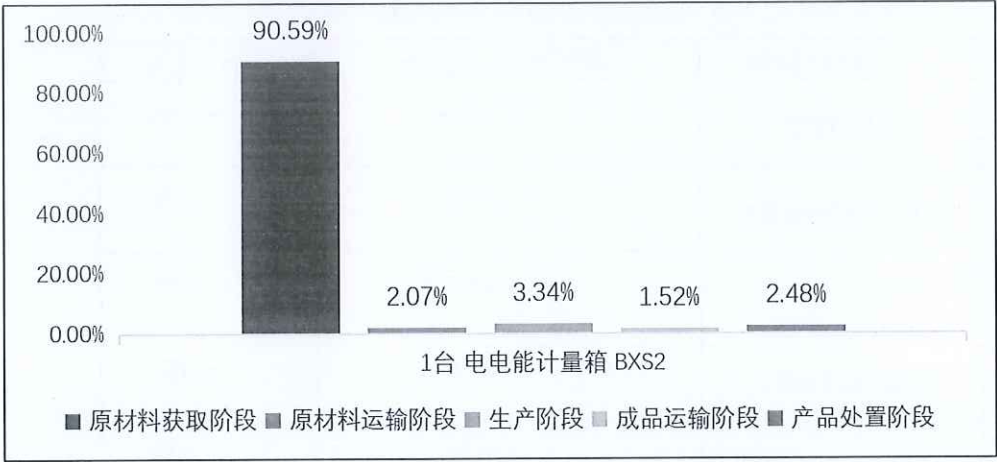
图 5.2-2-3 1 台 电能计量箱 BXS2 生命周期阶段碳排放分布图
