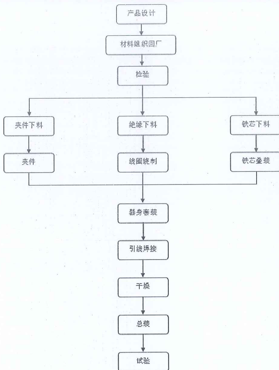
工艺流程图
