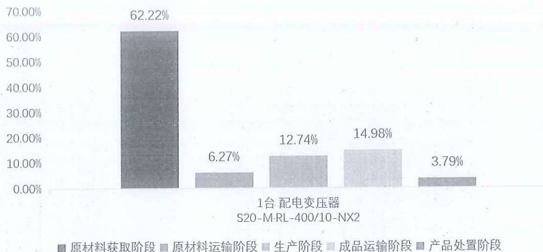
图 5.2.2 1 台配电变压器 S20-M • RL-400/10-NX2 (生命周期阶段碳排放分布图)
