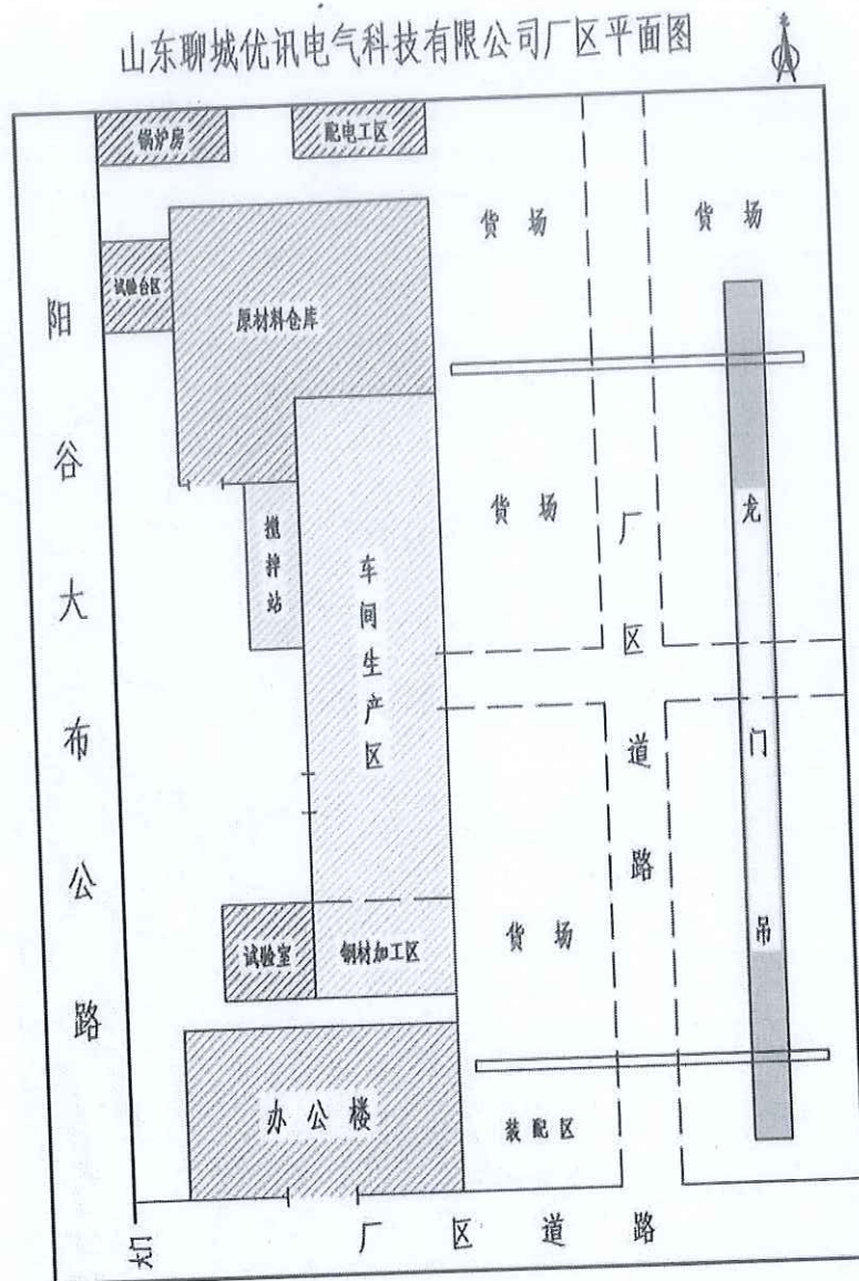
厂区平面图
