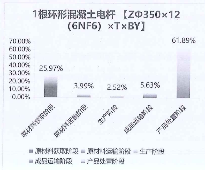
图 5.2-2 一根环形混凝土电杆【ZΦ350×12（6NF6）×T×BY】
