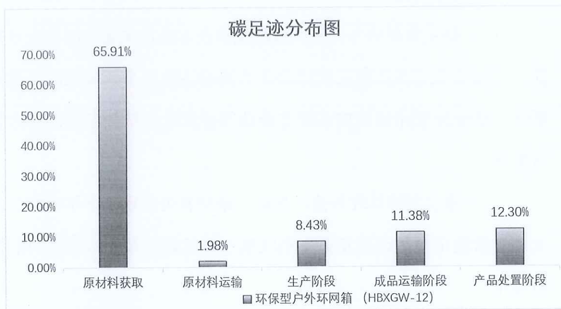
图 5.2.1.2 环保型户外环网箱 (HBXGW-12) 生命周期阶段碳排放分布图
