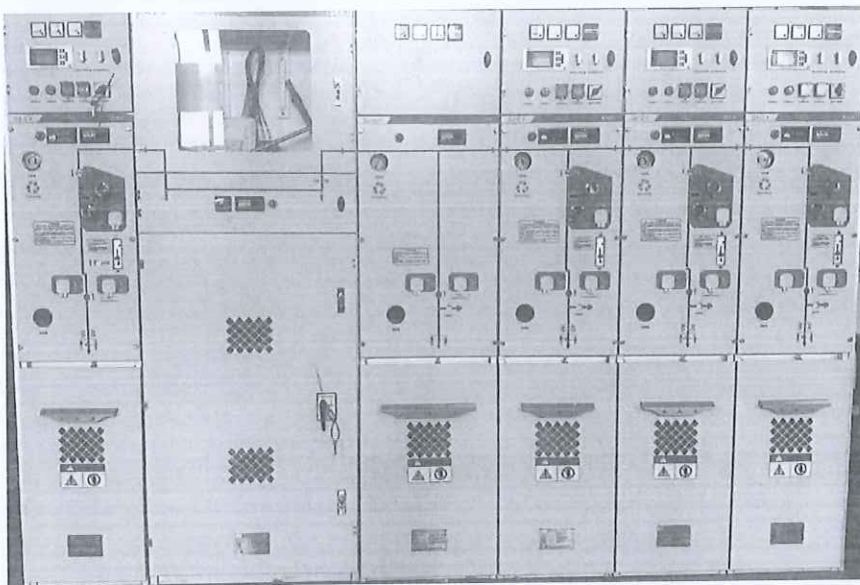
环保型中压环网开关设备 (CLH-12(V)/630-20)
