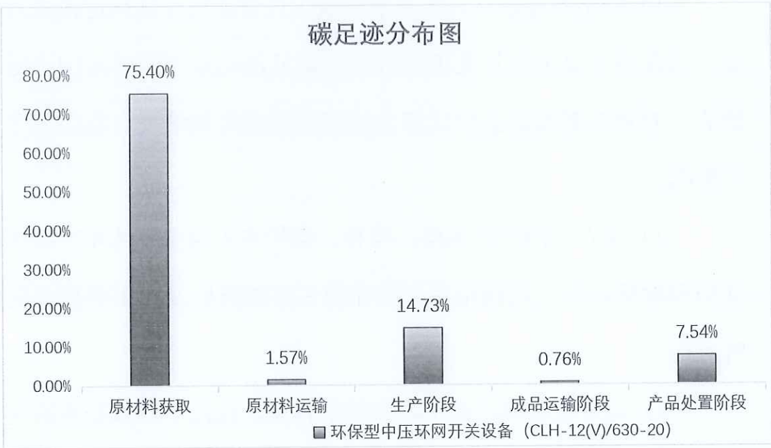
图 5.2.1.2 环保型中压环网开关设备 (CLH-12(V)/630-20) 生命周期阶段碳排放分布
