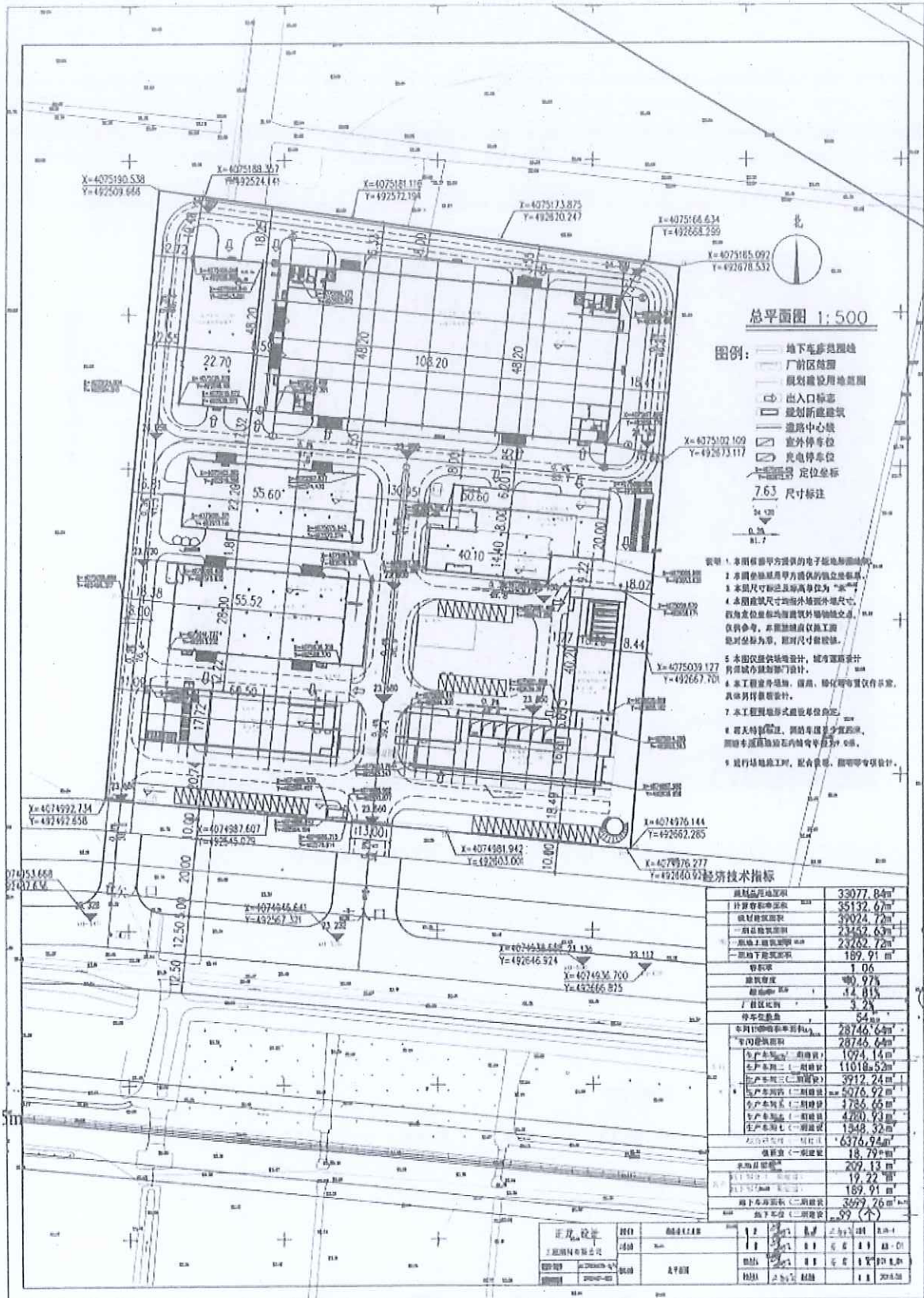
厂区平面图
