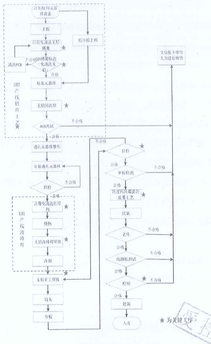
IFT 智能融合终端板卡焊接生产流程图
