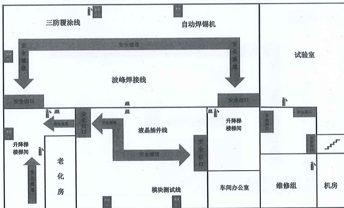
仙鹿车间二层
