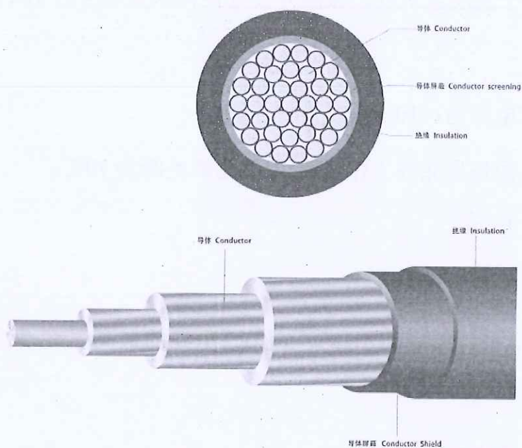
额定电压 10kV 铝芯交联聚乙烯绝缘架空电缆 (JKLYJ-10kV 1 \times 240\text{mm}^2 )
