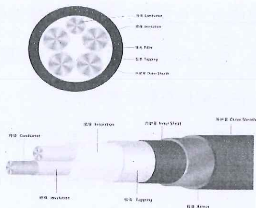
铜芯交联聚乙烯绝缘钢带铠装聚氯乙烯护套耐火电力电缆 (NH-YJV22 0.6/1kV 4× 240+1×120mm 2 )
