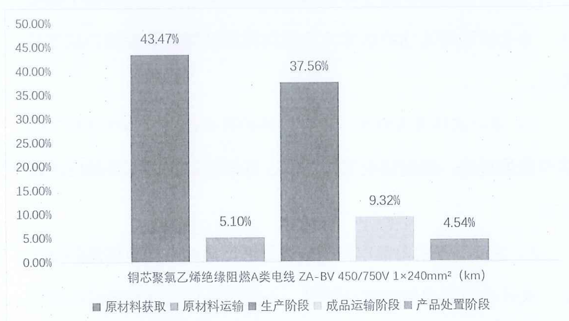
图 5.2.1-2 铜芯聚氯乙烯绝缘阻燃 A 类电线 ZA-BV 450/750V 1×240mm 2 生命周期阶段碳排放分布图
