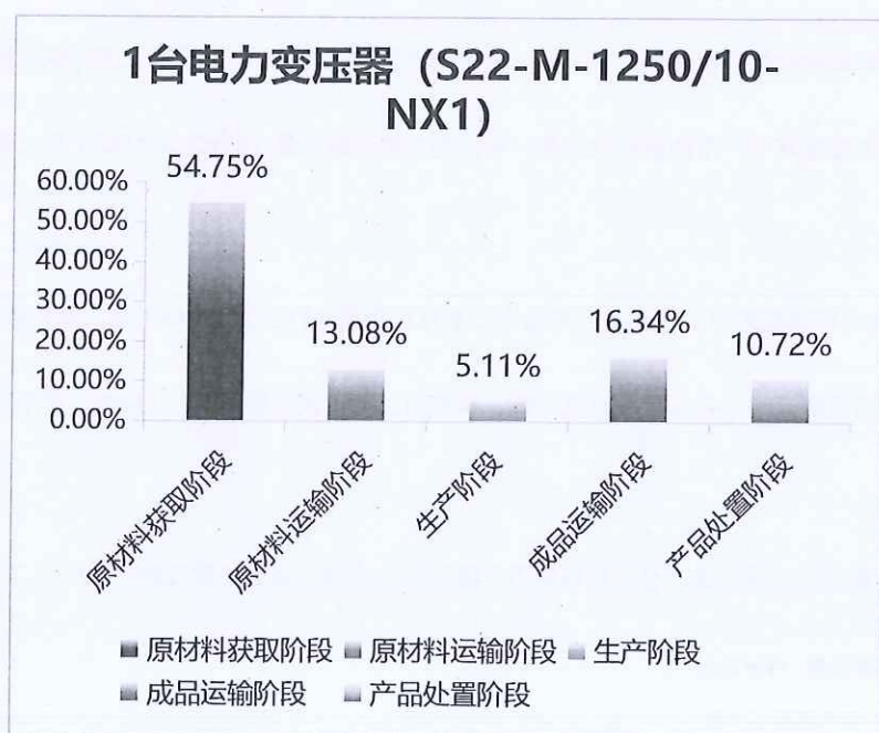
图 5.2-2 1 台电力变压器 (S22-M-1250/10-NX1)
