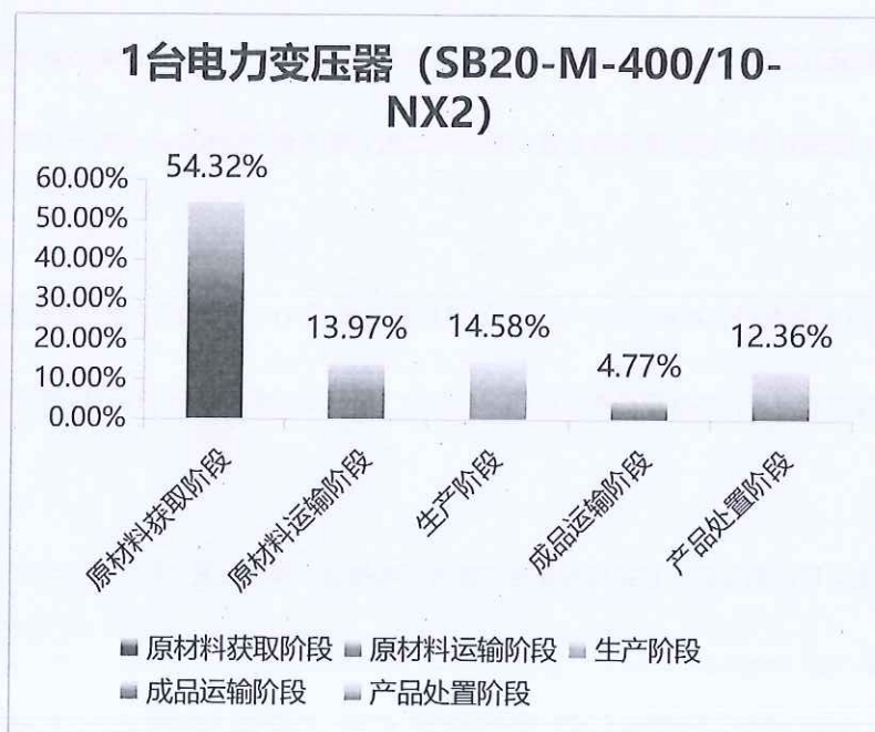
图 5.2-2 1 台电力变压器 (SB20-M-400/10-NX2)
