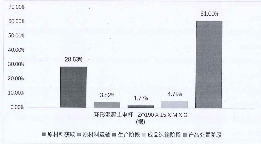
图 5.2.2 环形混凝土电杆 ZΦ190×15×M×G 生命周期阶段碳排放分布图
