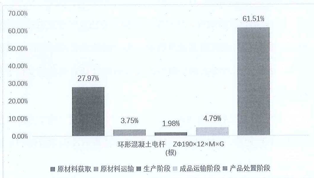
图 5.2.2 环形混凝土电杆 Z\Phi 190\times 12\times M\times G 生命周期阶段碳排放分布图
