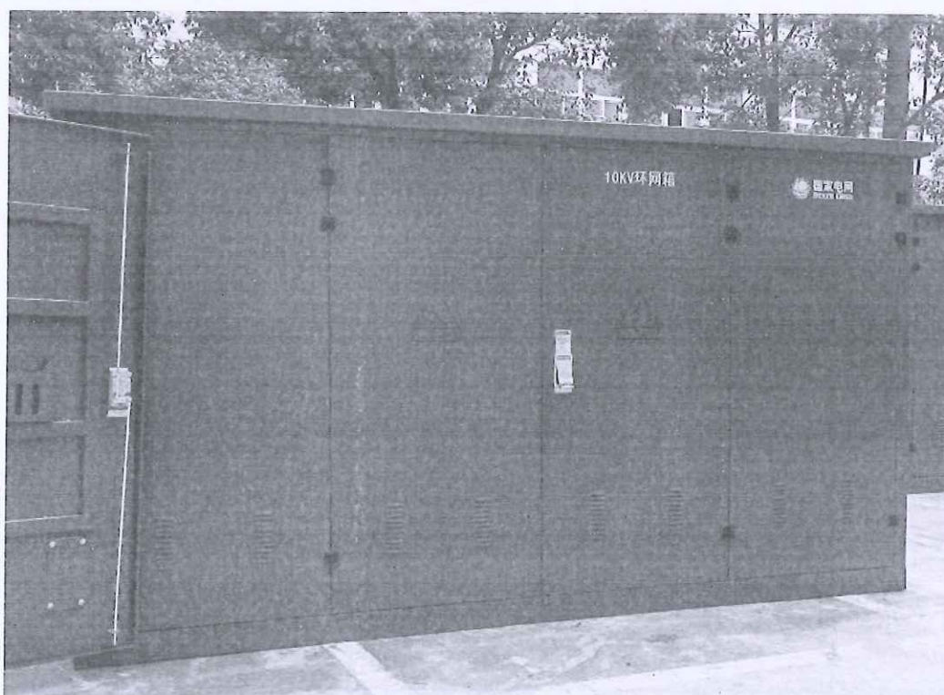
环网箱(开闭所) DHXGW-12 型
