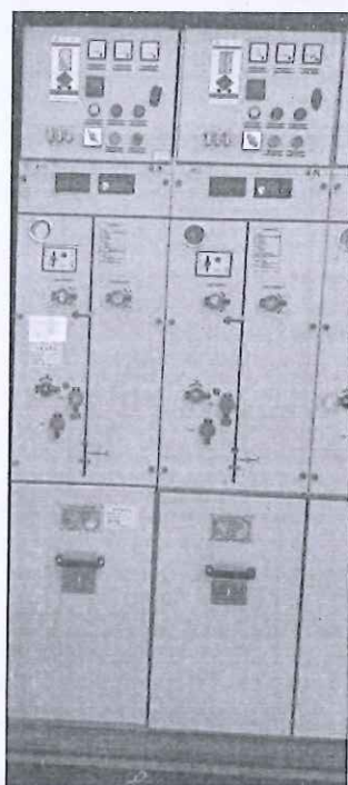
环保型中压环网开关设备 DHXGN-12(V)/630-20 型
