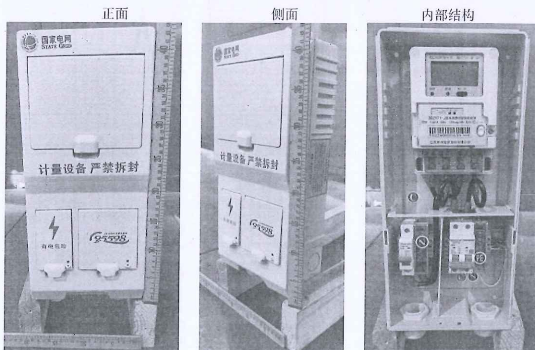
单相单表位非金属计量箱 PXD1
