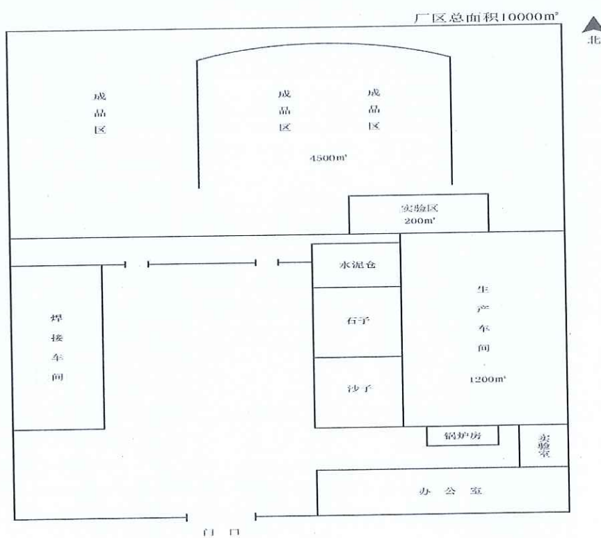
保定金昭水泥制品制造有限公司平面布置图
