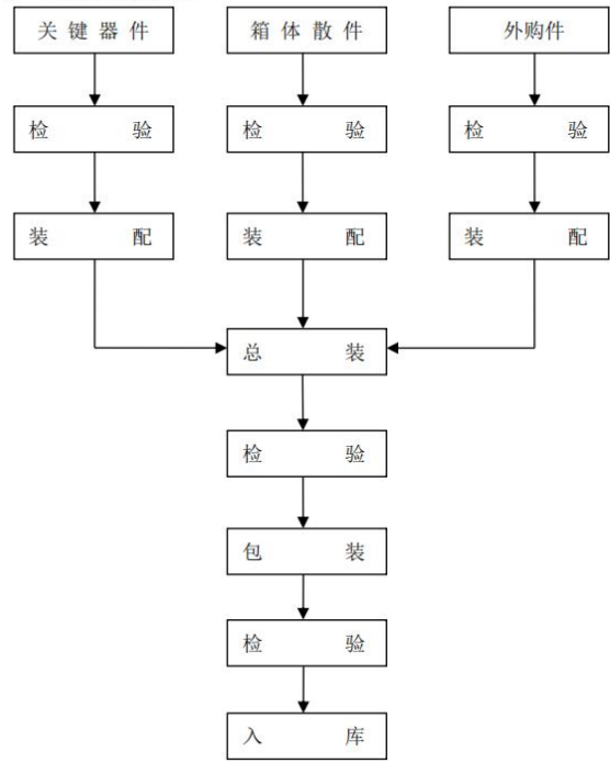
二、 装配工艺流程
