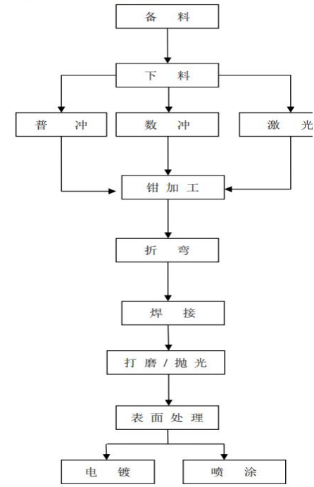
一、 钣金零件生产流程
