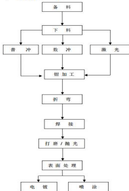
一、 钣金零件生产流程
