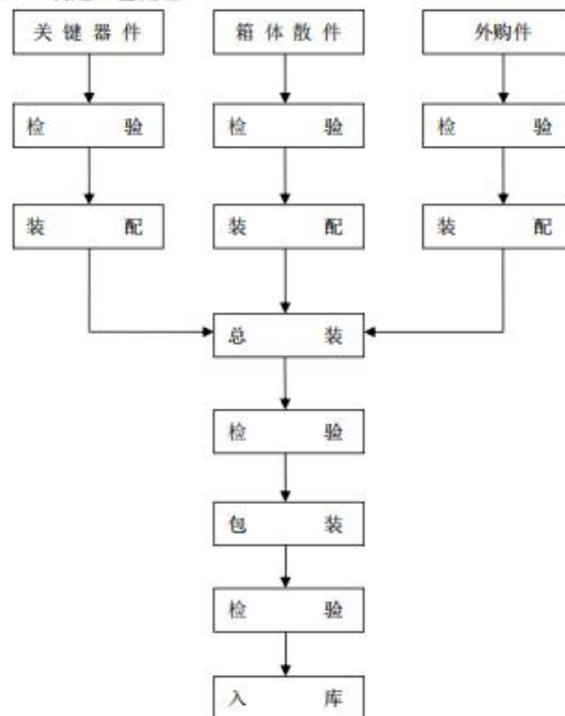
二、 装配工艺流程
