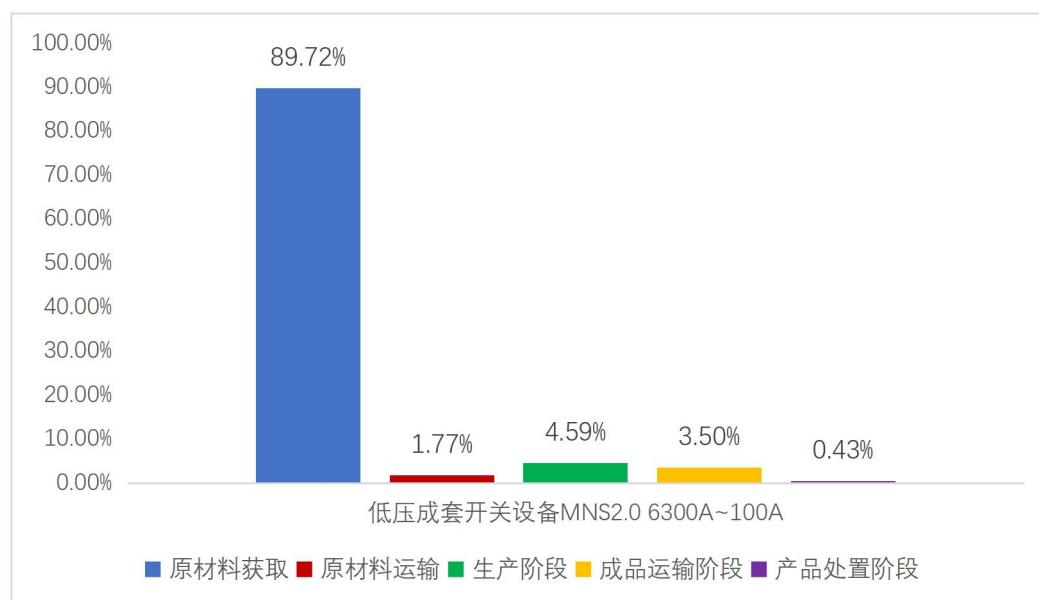
图 5.2-2 低压成套开关设备 MNS2.0 6300A~100A 生命周期阶段碳排放分布图
