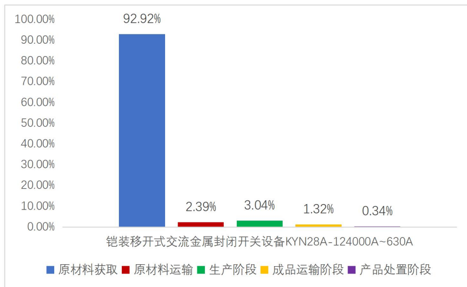
图 5.2-2 铠装移开式交流金属封闭开关设备 KYN28A-12 4000A~630A 生命周期阶段碳排放分布图
