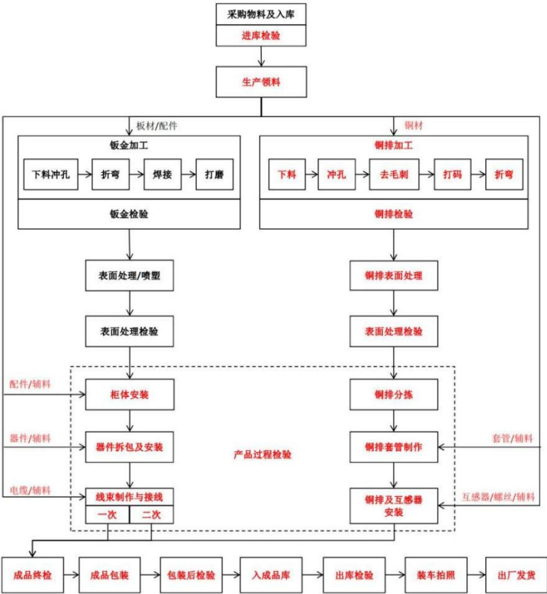
成套配电产品生产工艺流程图
