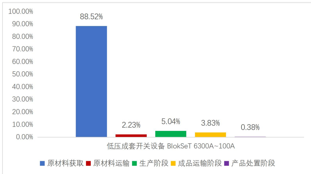
图 5.2-2 低压成套开关设备 BlokSeT 6300A~100A 生命周期阶段碳排放分布图
