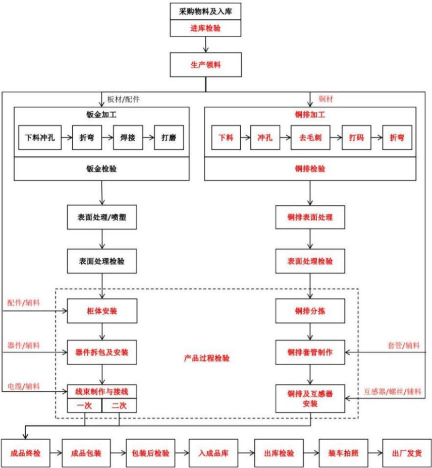
成套配电产品生产工艺流程图
