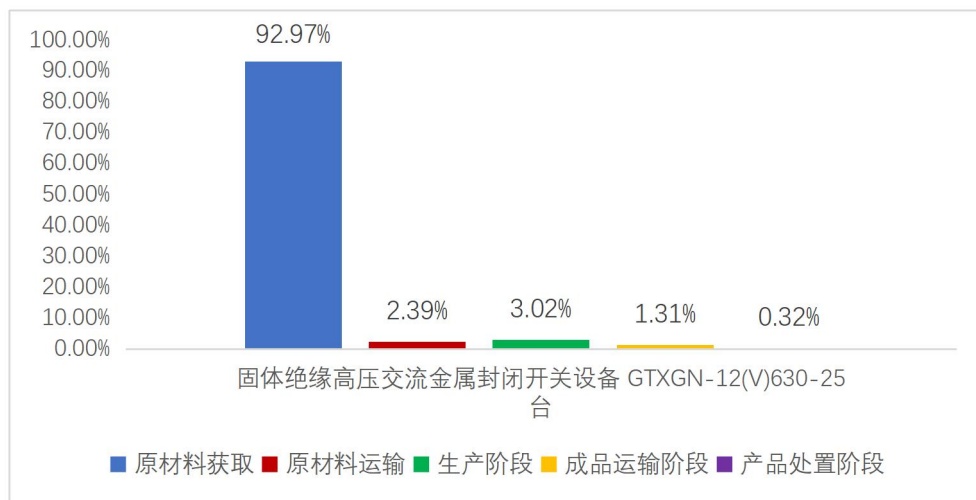
图 5.2-2 铠装移开式交流金属封闭开关设备 MVnex-12 4000A~630A 生命周期阶段碳排放分布图
