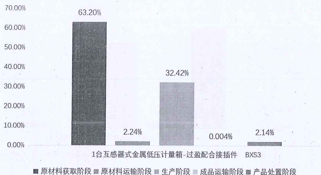
图 5.2-20 生命周期阶段碳排放分布图
