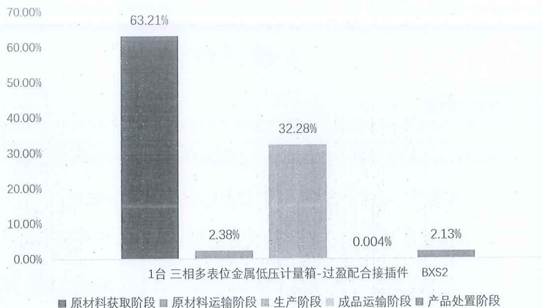
图 5.2-22 生命周期阶段碳排放分布图
