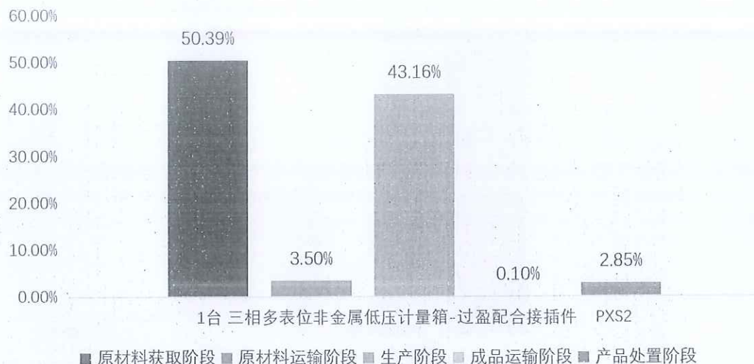
图 5.2-18 生命周期阶段碳排放分布图
