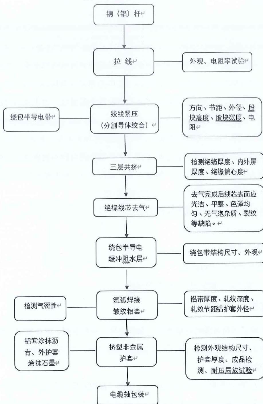
110kV 电力电缆生产工艺流程图
