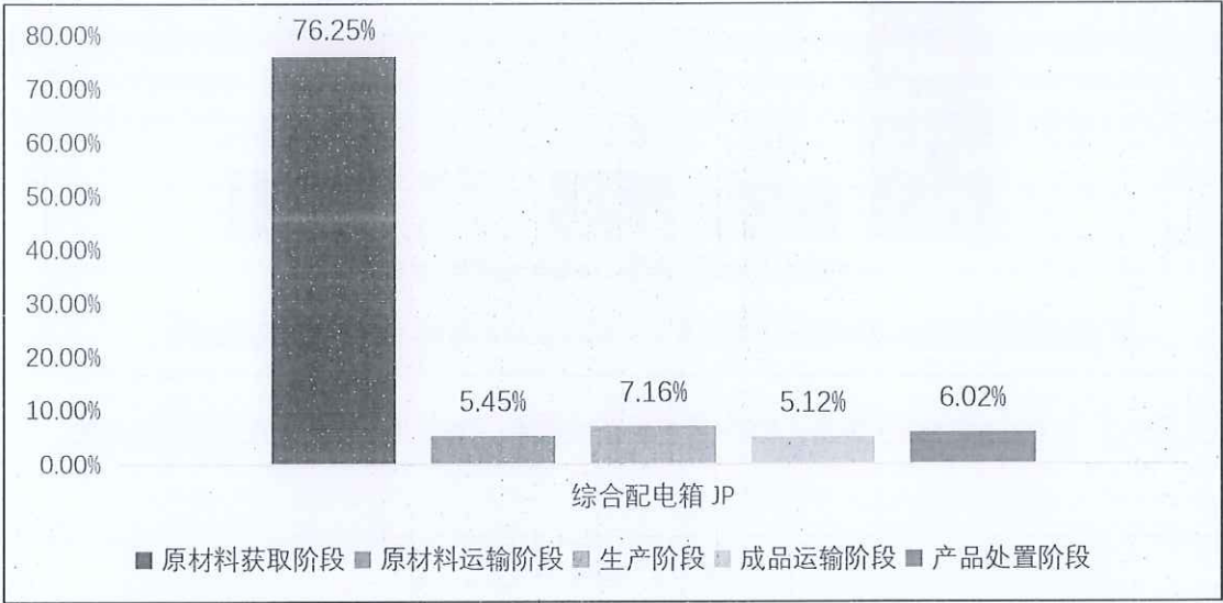
图 5.2-2-2 1 台 综合配电箱 JP 生命周期阶段碳排放分布图
