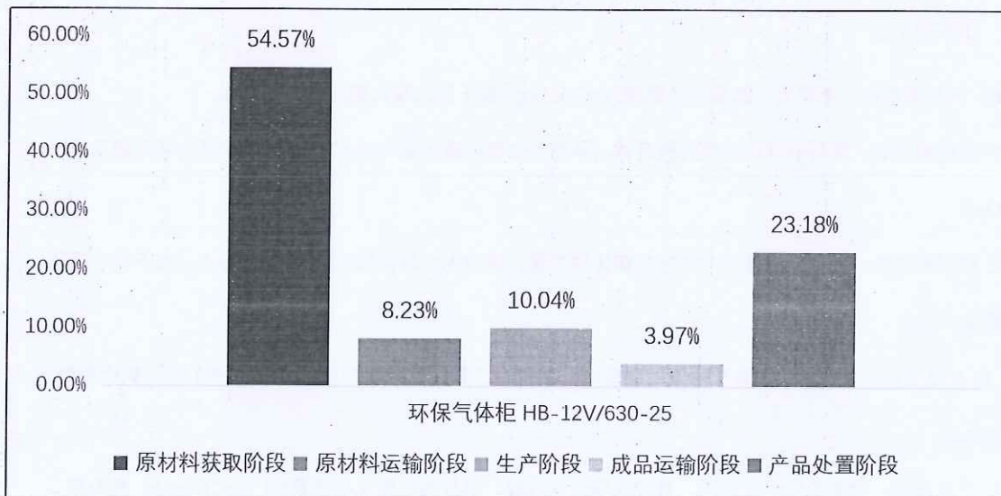
图 5.2-2-1 1 台 环保气体柜 HB-12V/630-25 生命周期阶段碳排放分布图
