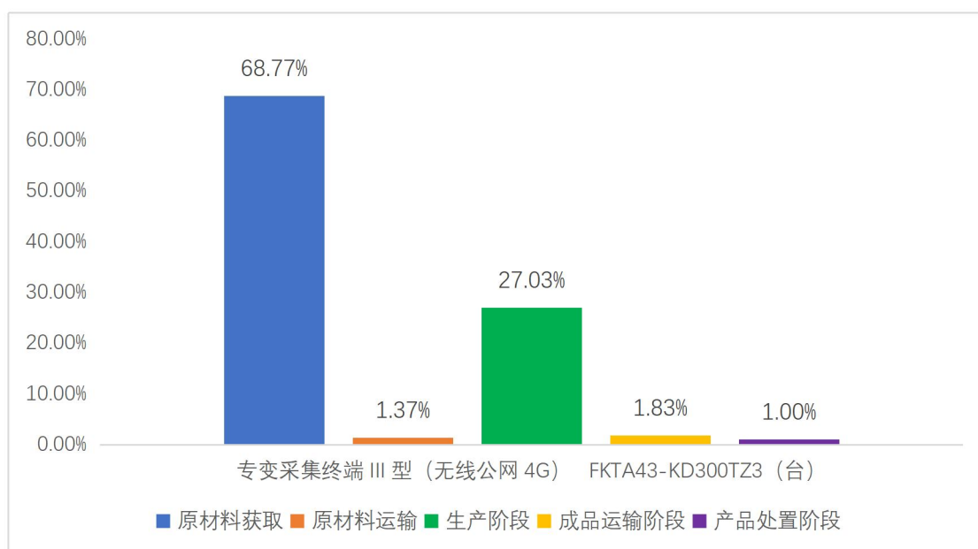
图 5.2.2 专变采集终端 III 型（无线公网 4G）FKTA43-KD300TZ3 生命周期阶段碳排放分布图
