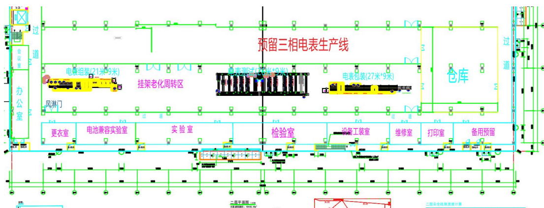
厂区平面图
