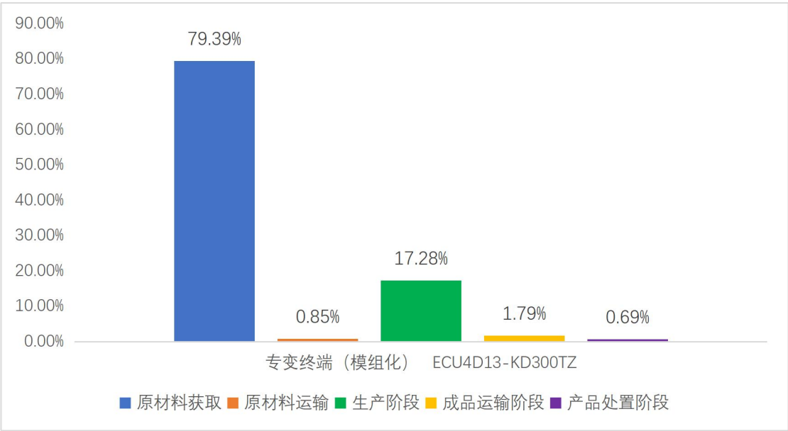
图 5.2.2 专变终端（模组化）（ECU4D13-KD300TZ）生命周期阶段碳排放分布图
