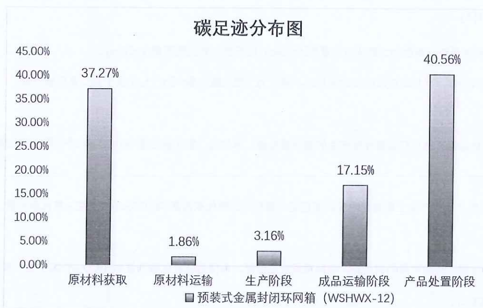
图 5.2.1.2 预装式金属封闭环网箱 (WSHWX-12) 生命周期阶段碳排放分布图
